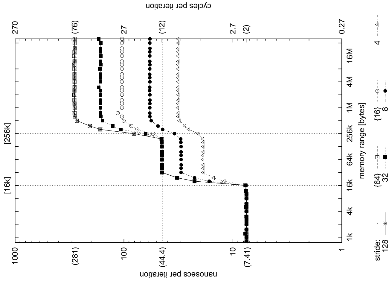
kamille.270.cache
